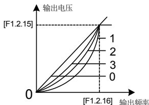
图 7-26 V/F 曲线
