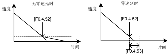
图 7-23 有无零速延时对比图
