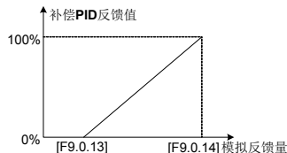
图 7-66 补偿 PID 反馈值定义示意图
