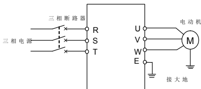
图 5-3 SVC 模式运行接线
