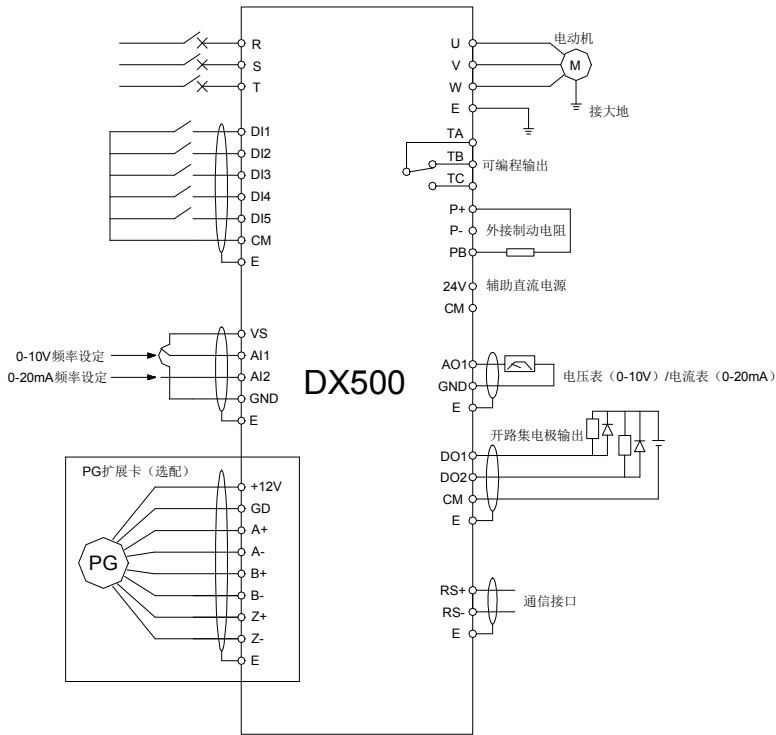
图 4-2 DX500 系列变频器基本接线
