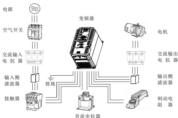
图 4-2 变频器的配线
