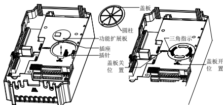
图 3-7-A I 类功能板的安装拆卸示意图
