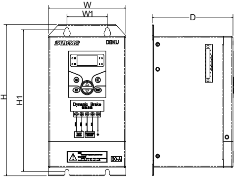
图 12-16 安装尺寸
