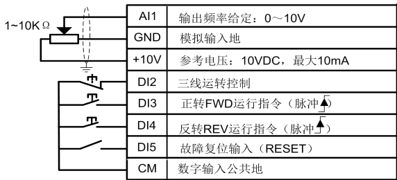
图 7-3 三线控制一/AI1 设定接线图
