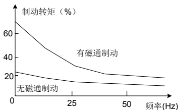
图 7-43 磁通制动曲线
