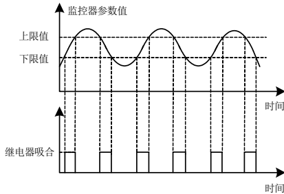
图 7-34-C 监控器功能示意图 3
