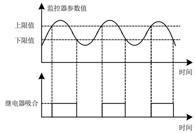
图 7-34-B 监控器功能示意图 2
