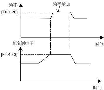
图 7-31-A 稳定运行过程的过压抑制
