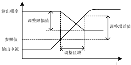
图 7-46 动平衡变量设置示意图
