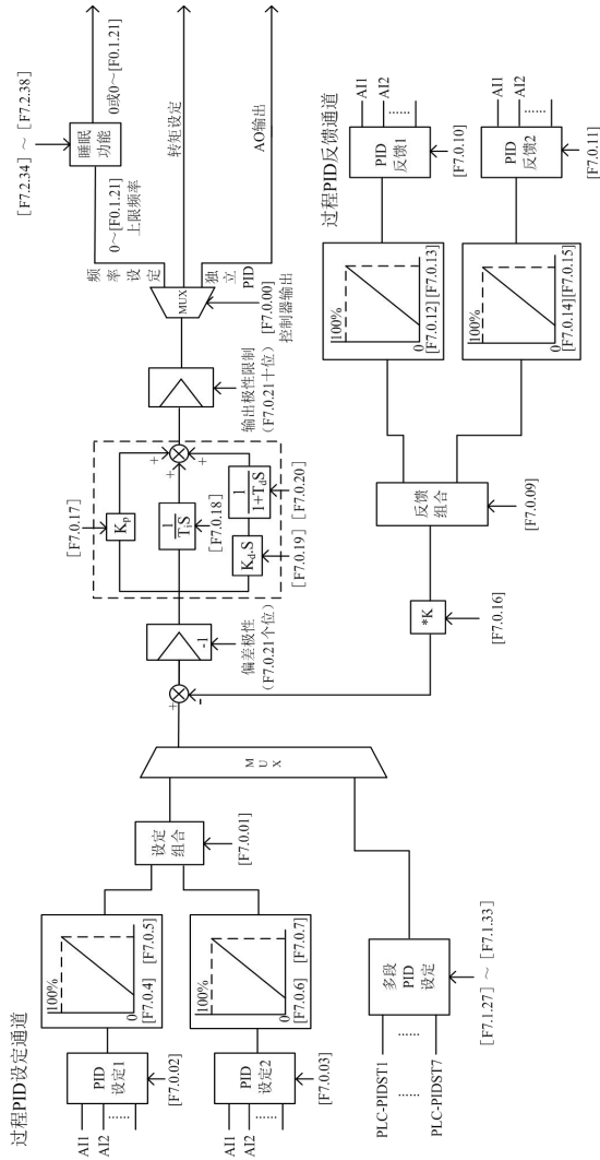
图 7-46 过程 PID 控制原理框图
