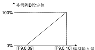
图 7-65 补偿 PID 设定值定义示意图
