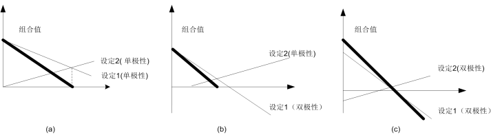
图 7-9-C 频率组合示意图 3
