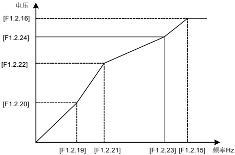
图 7-28 V/F 自定义曲线
