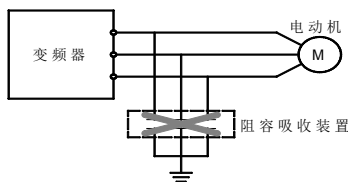
图 4-1 输出端禁止连接阻容吸收装置示意图
