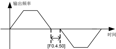
图 7-21 正反转过渡死区示意图
