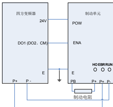
图 13-17 接线示意
