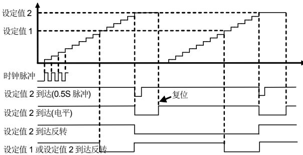
图 7-42-B 计数器功能 2
