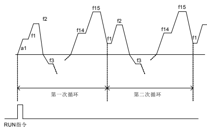
图 7-48-D 简易 PLC 运行连续循环模式
