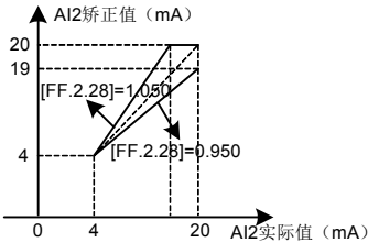
图 7-70-B AI2 增益矫正曲线
