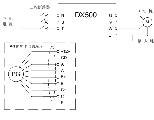
图 5-4 VC 模式运行接线
