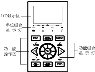
图 5-1-B 双行 LCD 标准操作面板
