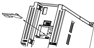
图 3-7-B II 类功能板的安装拆卸示意图
