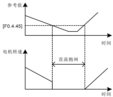
图 7-19 直流抱闸示意图
