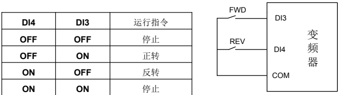
图 7-13-A 两线式运行模式 1
