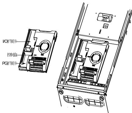
图 3-6 扩展卡的拆卸安装示意图
