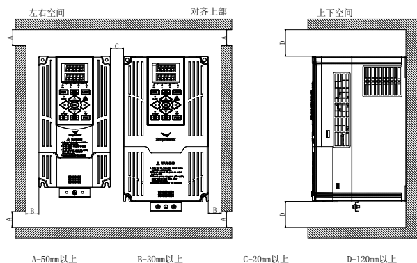
图 3-2 两台变频器（4.0KW 以上）左右安装尺寸
