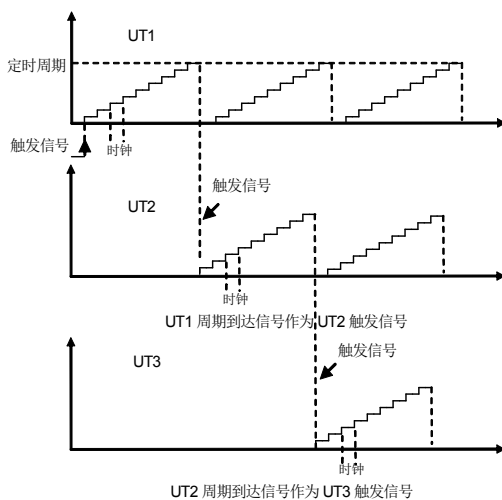
图 7-41-E 定时器 (UT1、UT2、UT3) 的触发串接功能
