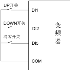
图 7-12 端子 UP/DW 接线示意图
