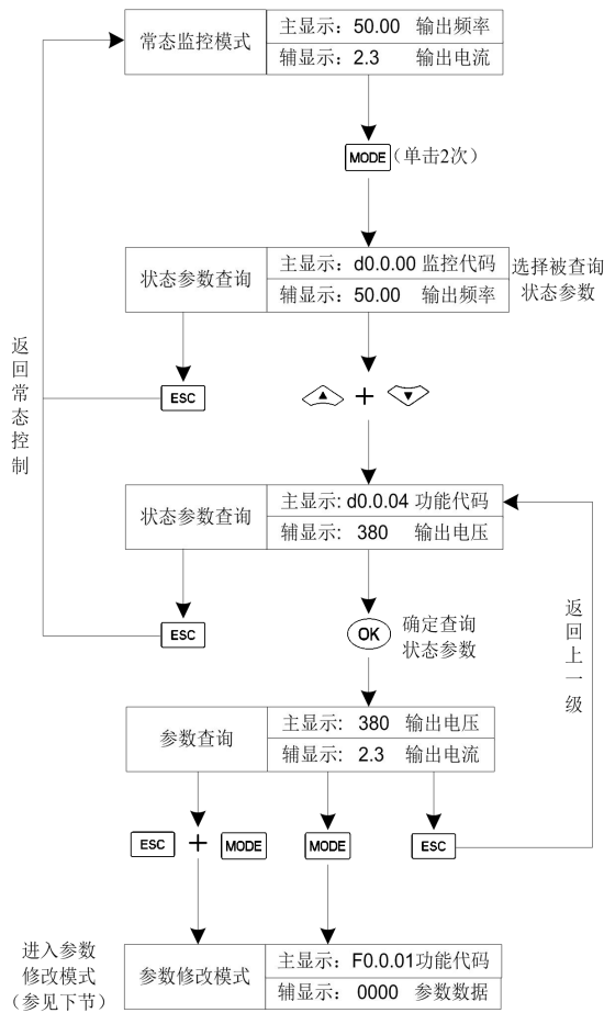
图 5-2 状态参数查询示意图
