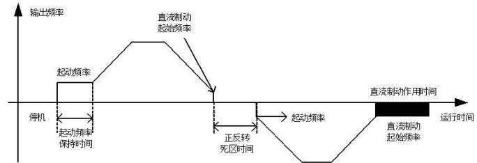
图 7-20 停机直流制动示意图
