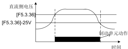
图 7-44 能耗制动
