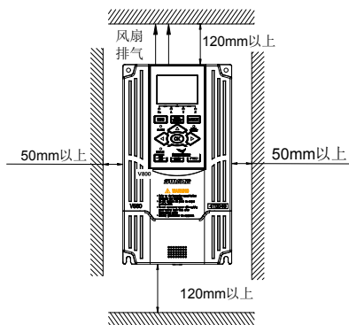
图 3-1-A 安装的间隔距离(30KW 及以下)
