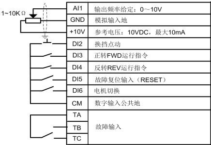
图 7-4 机床主轴驱动宏 AI1 设定接线图
