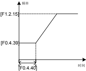
图 7-17 起动频率示意图
