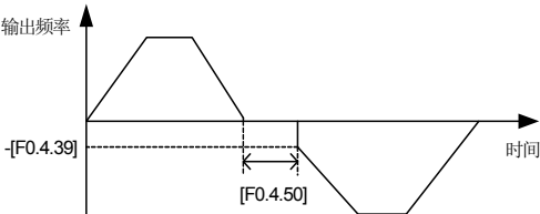
图 7-22 起动频率正反转切换示意图
