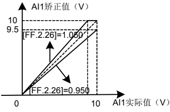
图 7-69-B AI1 增益矫正曲线
