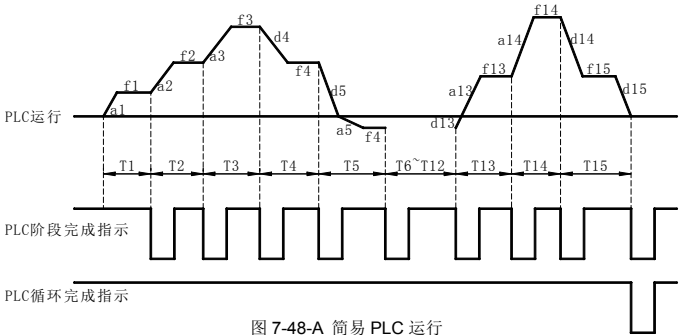
图 7-48-A 简易 PLC 运行
