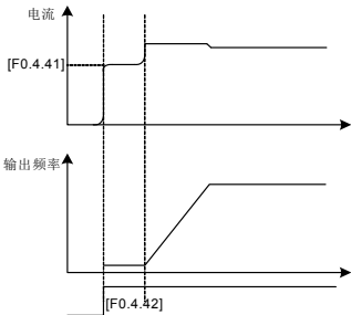
图 7-18 起动预励磁输出
