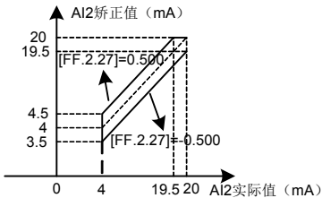
图 7-70-A AI2 零偏矫正曲线
