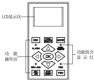
图 5-1-A 小 LCD 面板
