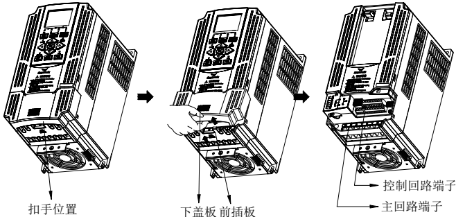
图 3-4 塑壳盖板的拆卸安装示意图
