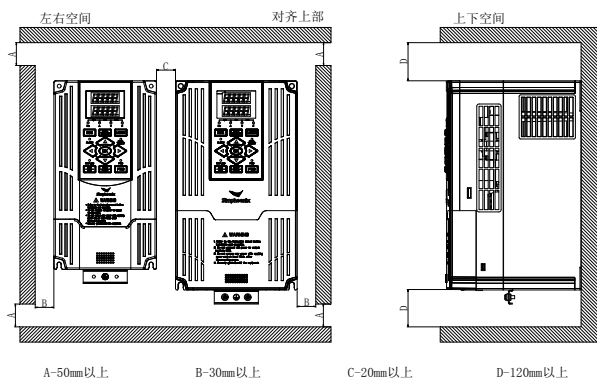
图 3-2 两台变频器（4.0KW 以上）左右安装尺寸
