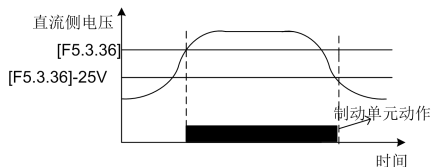
图 7-44 能耗制动
