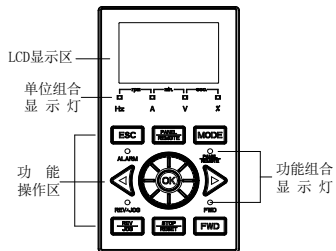
图 5-1-B 双行 LCD 标准操作面板
