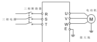
图 5-3 SVC 模式运行接线
