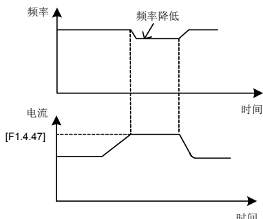
图 7-32-B 限流调节示意图
