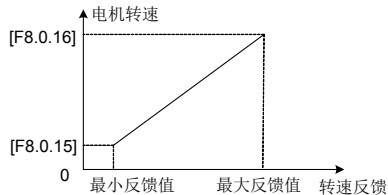
图 7-62 转速反馈值和电机转速对应关系图
