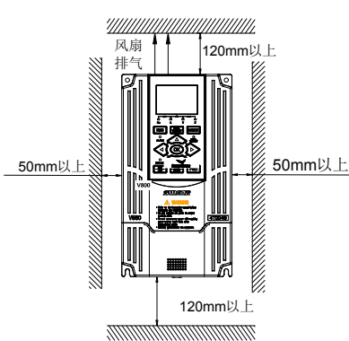
图 3-1-A 安装的间隔距离(30KW 及以下)
