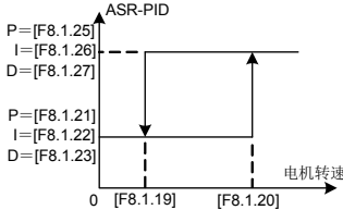
图 7-63-A 双 PID 参数 (滞环切换)
