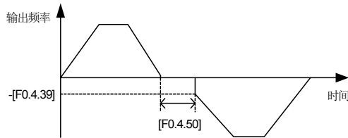
图 7-22 起动频率正反转切换示意图
