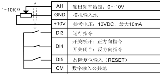
图 7-2-B 两线控制二 AI1 设定接线图
