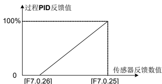
图 7-58 反馈百分比与对应传感器数值的的关系曲线
