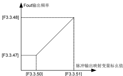
图 7-35 脉冲输出 Fout 特性曲线
