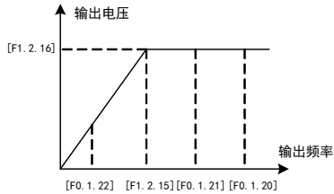
图 7-10 频率参数定义示意图
