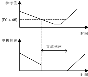
图 7-19 直流抱闸示意图
