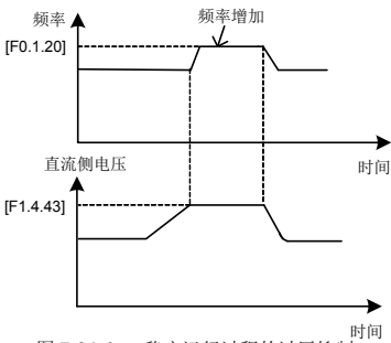
图 7-31-A 稳定运行过程的过压抑制
