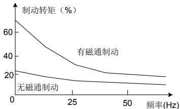
图 7-43 磁通制动曲线
