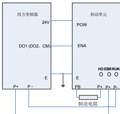
图 13-17 接线示意
