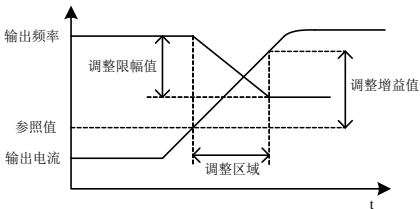
图 7-46 动平衡变量设置示意图
