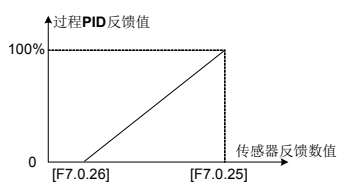
图 7-58 反馈百分比与对应传感器数值的范围曲线
