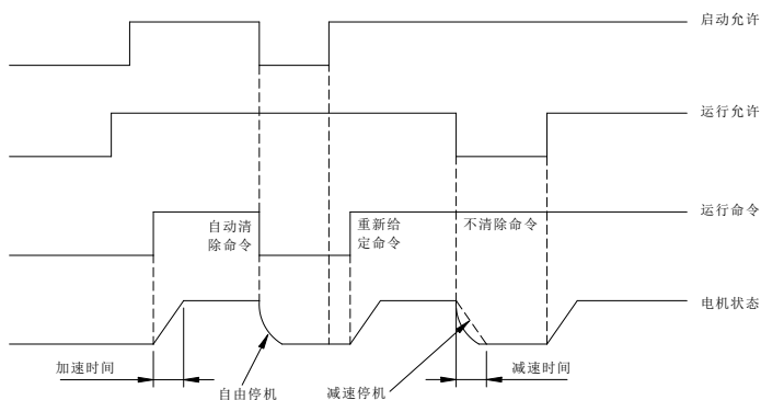
图 7-15 起动过程原理图
