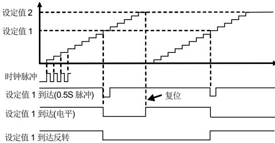
图 7-42-A 计数器功能 1
