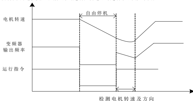
图 7-16 转速跟踪起动示意图
