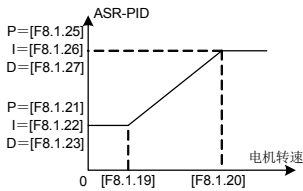
图 7-63-B 双 PID 参数（连续切换）
