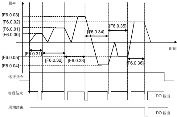
图 7-48-C 简易 PLC 运行单循环停机模式
