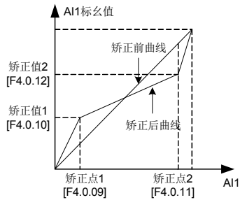
图 7-38 模拟输入 AI1 曲线矫
