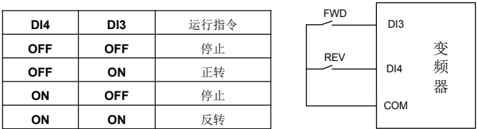
图 7-13-B 两线式运行模式 2
