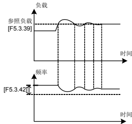
图 7-45 负载动平衡功能示意图
