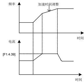
图 7-30 加/减速电流限制示意图
