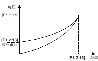
图 7-27-A 降转矩曲线转矩提升示意图
