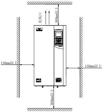
图 3-1-B 安装的间隔距离(37KW 及以上)
