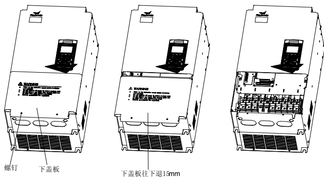
图 3-4 钣金盖板的拆卸安装示意图
