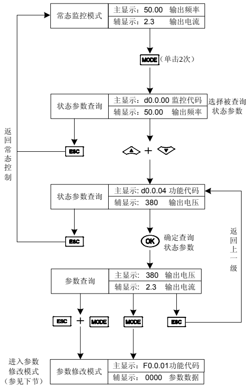
图 5-2 状态参数查询示意图
