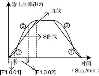
图7-21 加减速曲线
