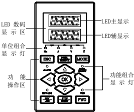
图 5-1-A 双行 LED 小面板 E580-4T0040G/4T0055P 及以下机型标配
