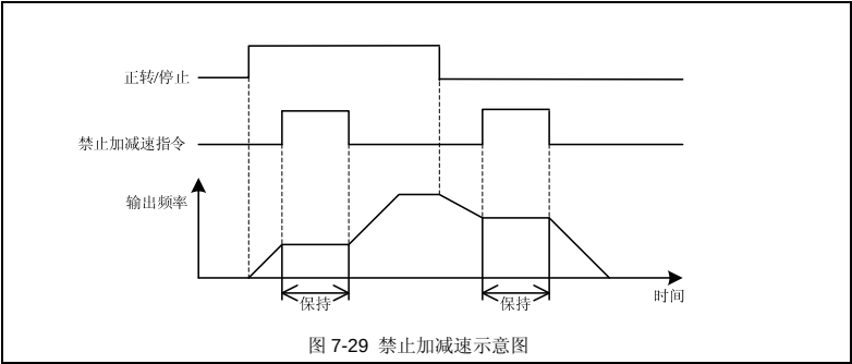
图 7-29 禁止加减速示意图
