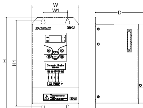
图 12-3 安装尺寸图
