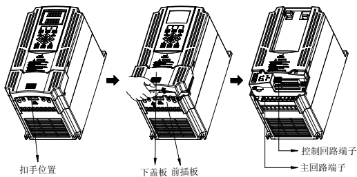
图 3-3 塑壳盖板的拆卸安装示意图
