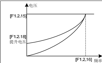
图 7-23-A 降转矩曲线转矩提升示意图
