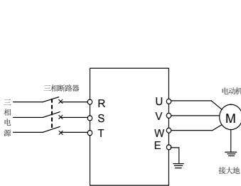
图 5-3 SVC 运行接线
