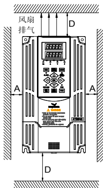
图 3-1 安装的间隔距离
