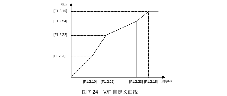
图 7-24 V/F 自定义曲线
