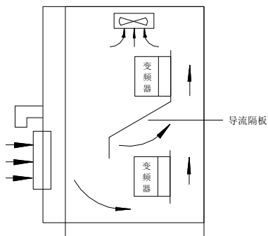
图 3-2 多台变频器（4.0KW 以上）上下安装尺寸
