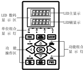
图 5-1-B 双行 LED 标准操作面板 E580-4T0055G/4T0075P 及以上机型标配
