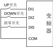
图 7-9 端子 UP/DW 接线示意图
