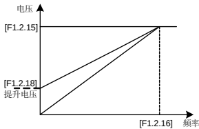
图 7-23-B 恒转矩曲线转矩提升示意图
