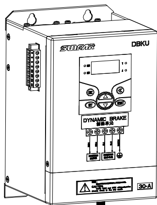
图 12-2 外观示意图
